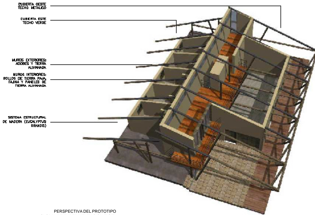
PERSPECTIVA DEL PROTOTIPO GLOBAL DE EXPERIMENTACION (PGE)
