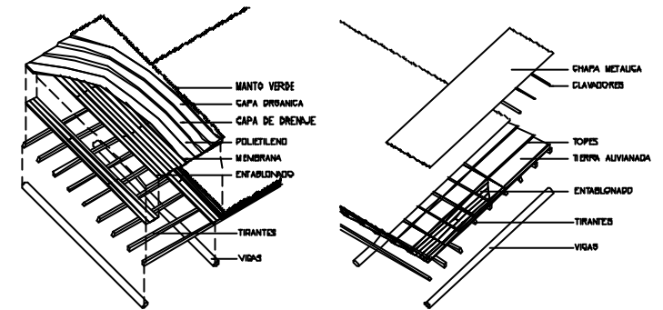
ISOMETRICAS DE TECHO VERDE Y TECHO METALICO
