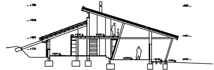
CORTE AA
